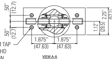
VIEW A-A
