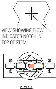
VIEW A-A
