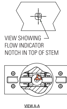
VIEW A-A
